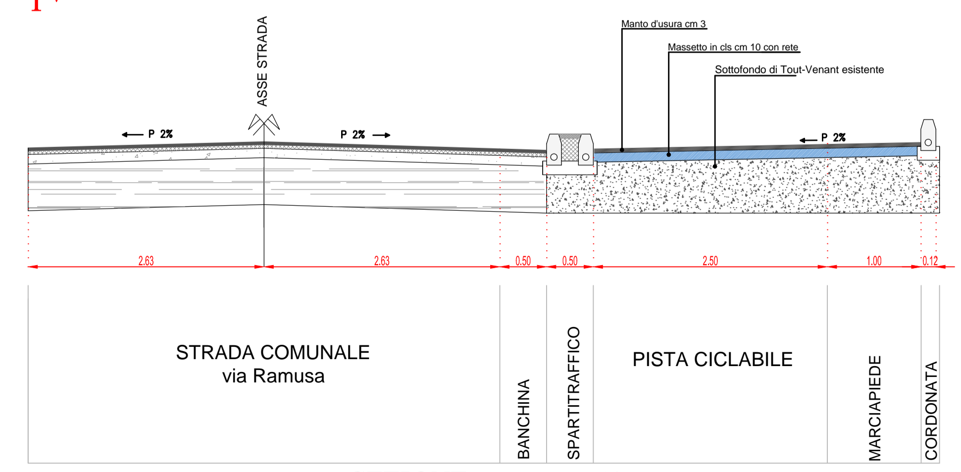
SEZIONE 1-1 sc 1:50
