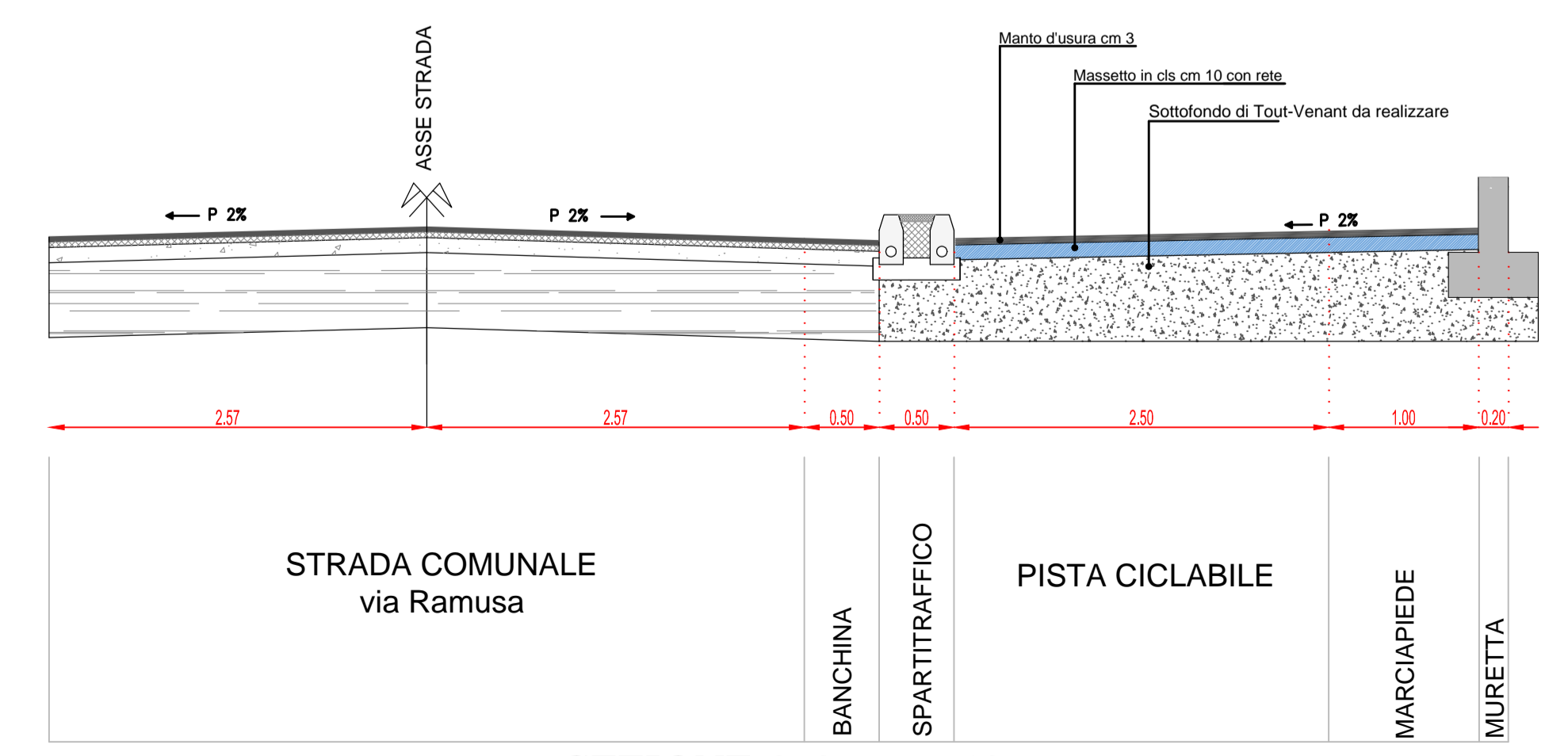
SEZIONE 2-2 sc 1:50
