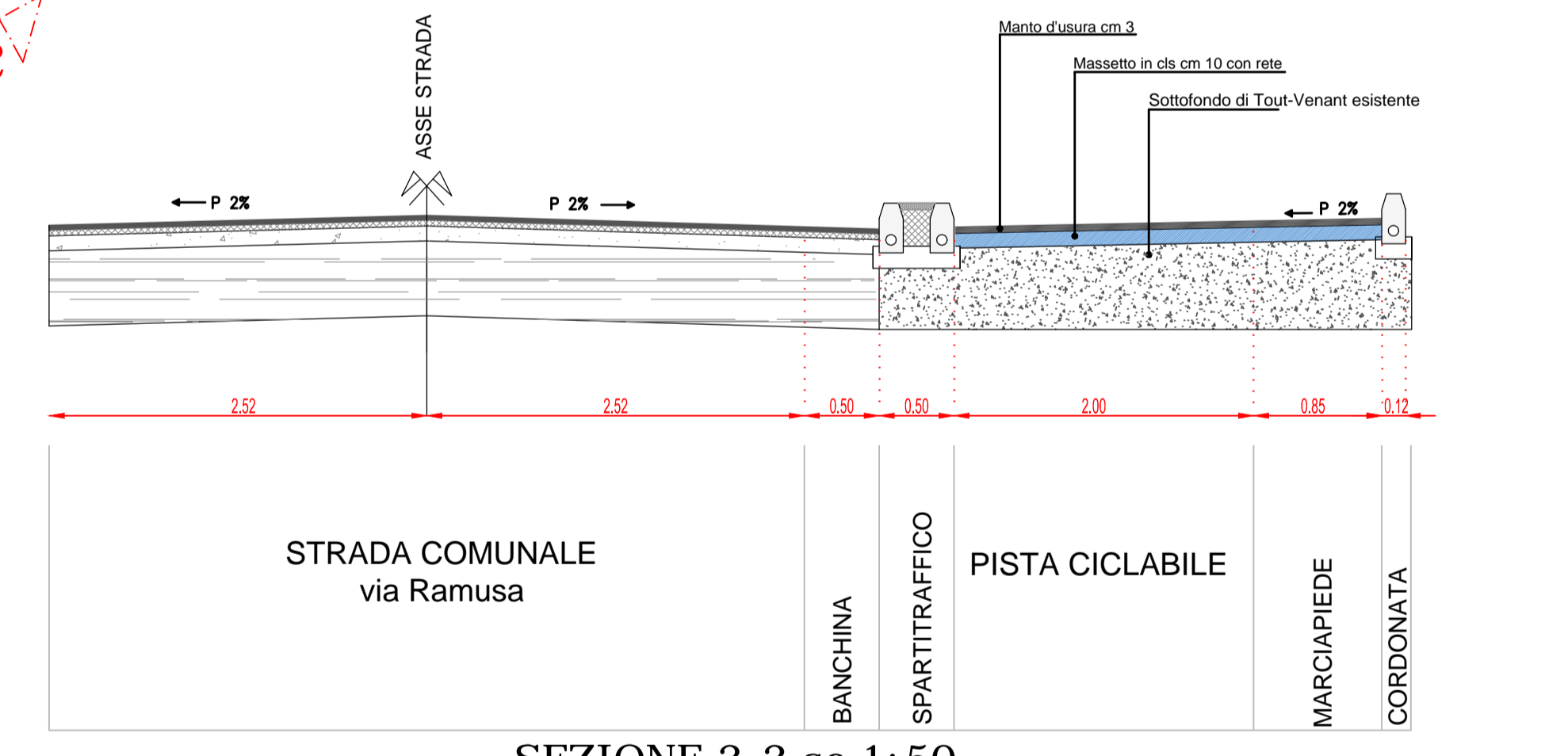
SEZIONE 3-3 sc 1:50
